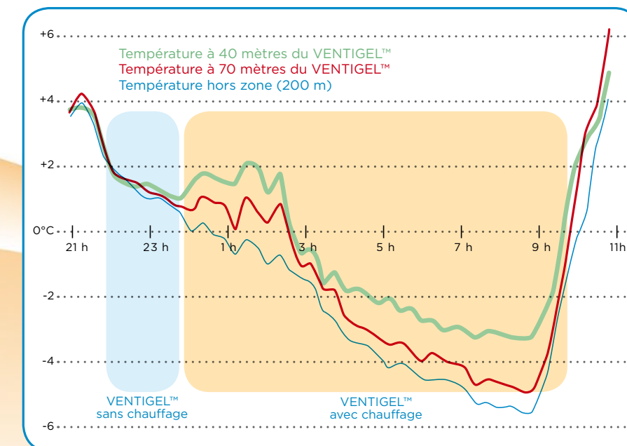
Relevé de température pendant une nuit de gel. VENTIGEL™ sans chauffage avant les températures négatives et avec chauffage dès que les températures descendent au dessous de 0°C
