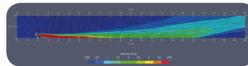
Simulations numériques des vitesses d'air du modèle V3b
