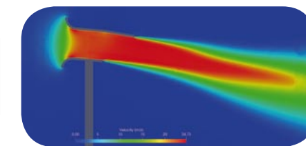
Simulations numériques des vitesses d'air du modèle V3b
